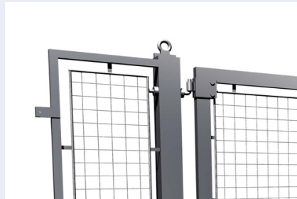
Løftering gjør det enkelt å flytte porten. Øyebolt M24. Hengsler M24.
